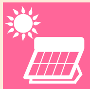
太陽熱利用
